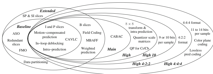
Fig. 12.11 H.264 profiles
